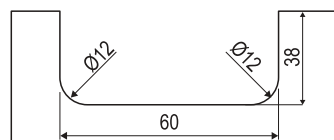
Dimenzije za pripremu (usecanje) stakla
