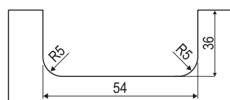
Dimenzije za pripremu (usecanje) stakla
