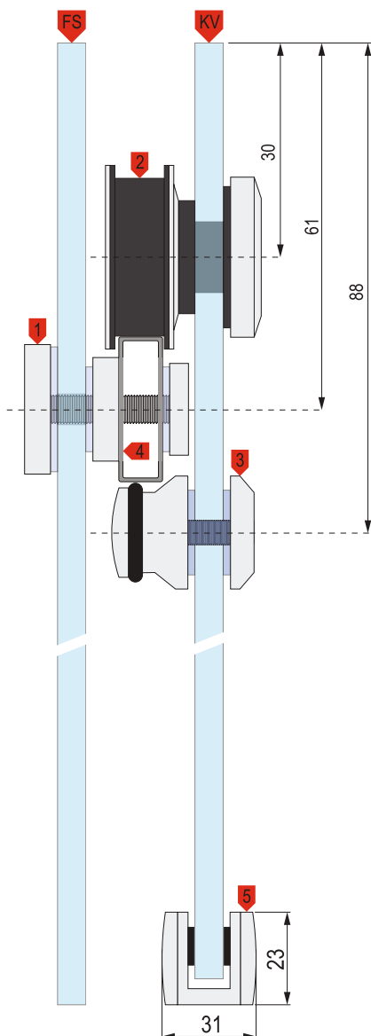
Bočni prikaz montaže kliznog sistema
