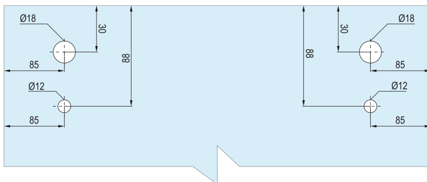
Priprema staklene ispune za klizni mehanizam
