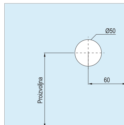
Priprema staklene ispune za ukopavajuću ručicu
