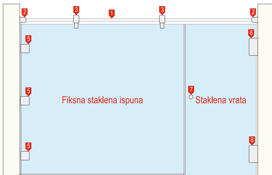
Pogled sa prednje strane (frontalno)
